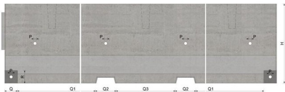
Prospetto laterale
