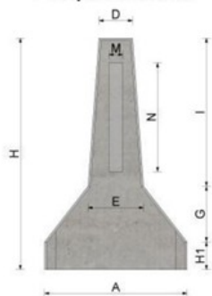
Prospetto frontale
