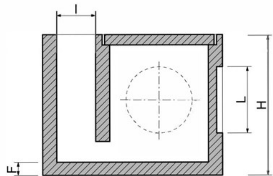
Sezione A-A
