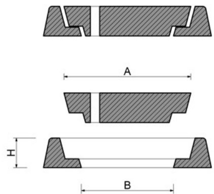
Sezioni A-A cod. 710-711-712
